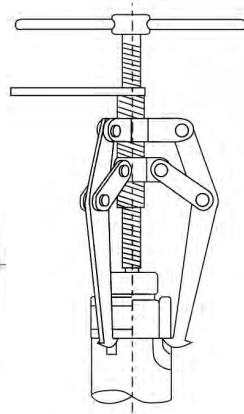
Извлечение внутреннего кольца с помощью инструментов для демонтажа
